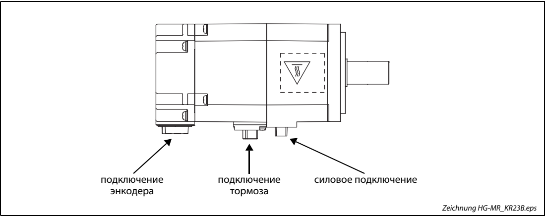
Рис. 3-4: Серводвигатели серий HG-MR и HG-KR
