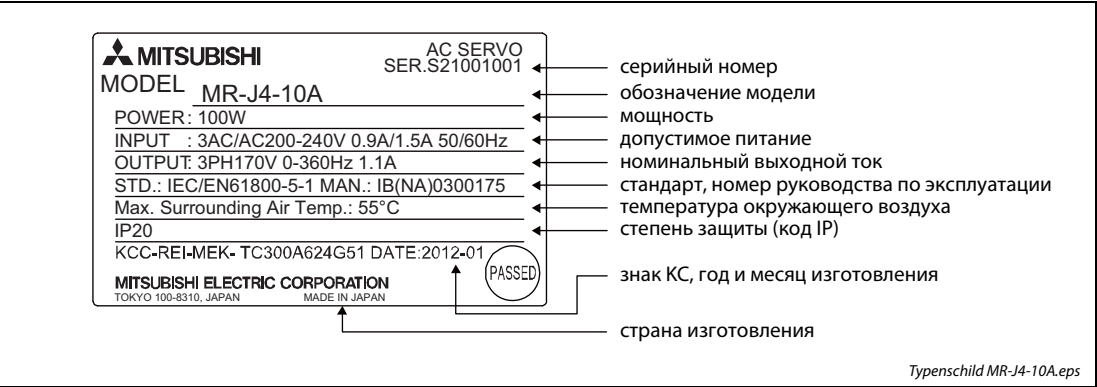
Рис. 2-12: Табличка данных MR-J4-10A
