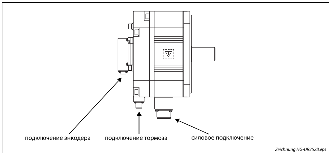
Рис. 3-12: Серводвигатели серии HG-UR
