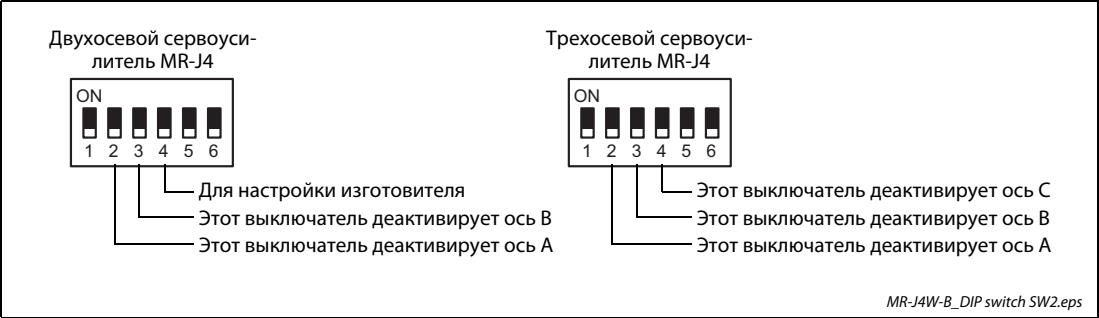
Рис. 4-21: Выключатели SW2-2, SW2-3 и SW2-4 для деактивации отдельных осей
