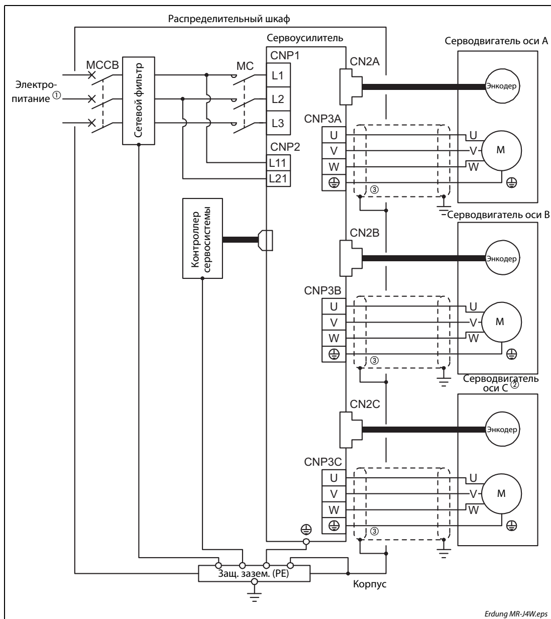
Рис. 4-23: Заземление сервоусилителя MR-J4W2-B или MR-J4W3-B
