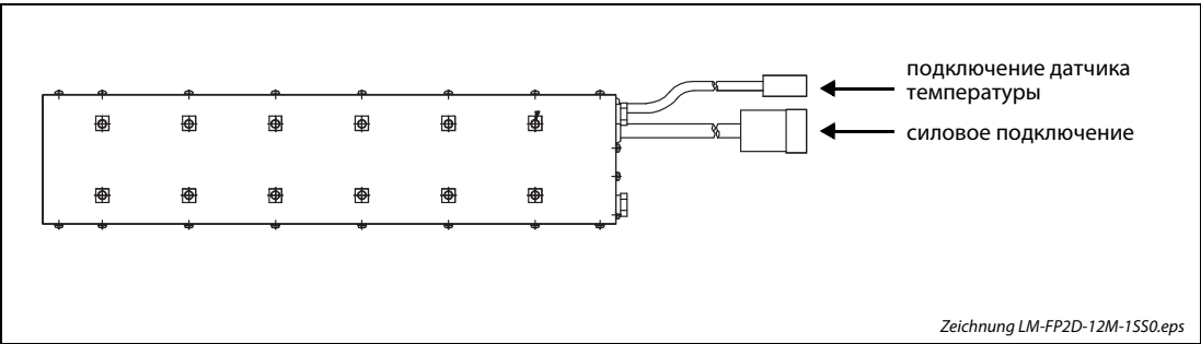
Рис. 3-21: Серводвигатели серии LM-F (первичный элемент – катушка)
