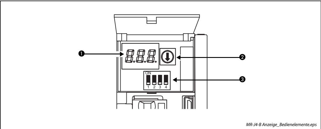
Рис. 6-14: Индикация и выключатели сервоусилителя MR-J4-B(-RJ)
