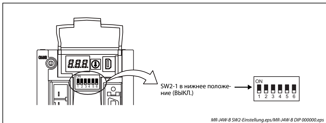
Рис. 6-26: Настройка выключателя SW2-1 для работы без серводвигателя с управлением с помощью контроллера
