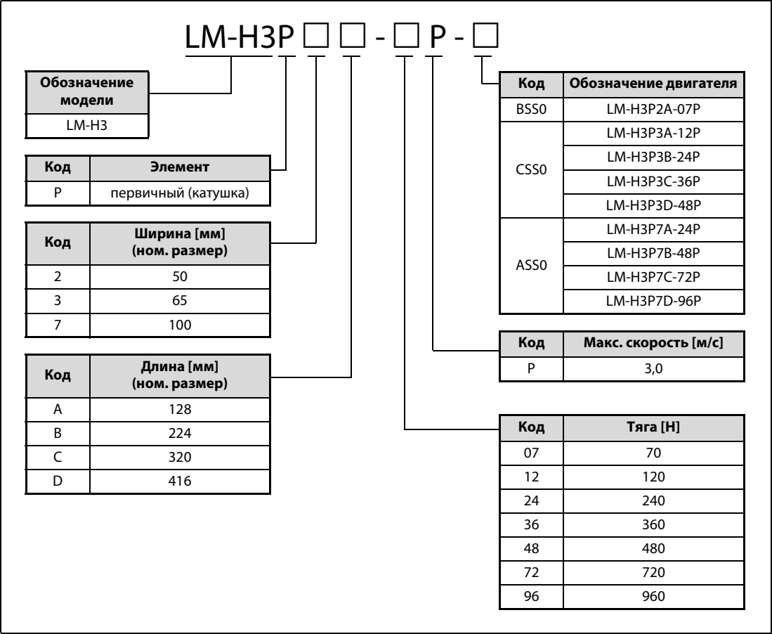
Рис. 3-15: Обозначение серводвигателей серий LM-H3 (первичный элемент – катушка)
