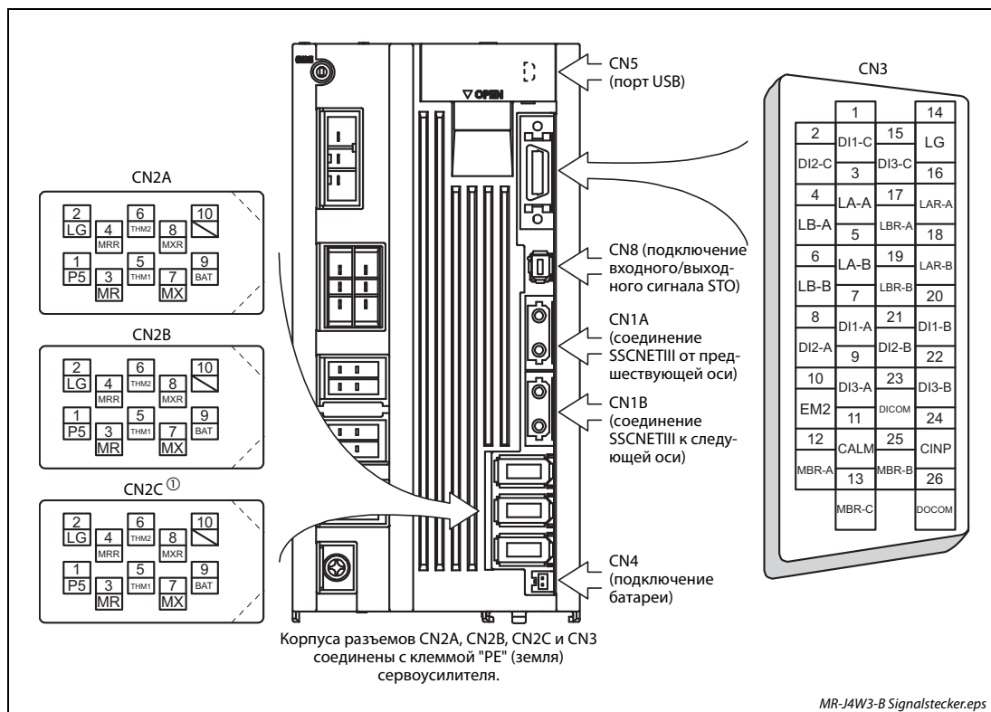
Рис. 4-5: Сигнальные выводы MR-J4W-B
