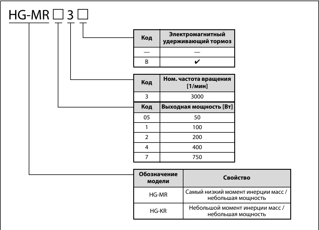
Рис. 3-3: Обозначение серводвигателей серий HG-MR и HG-KR
