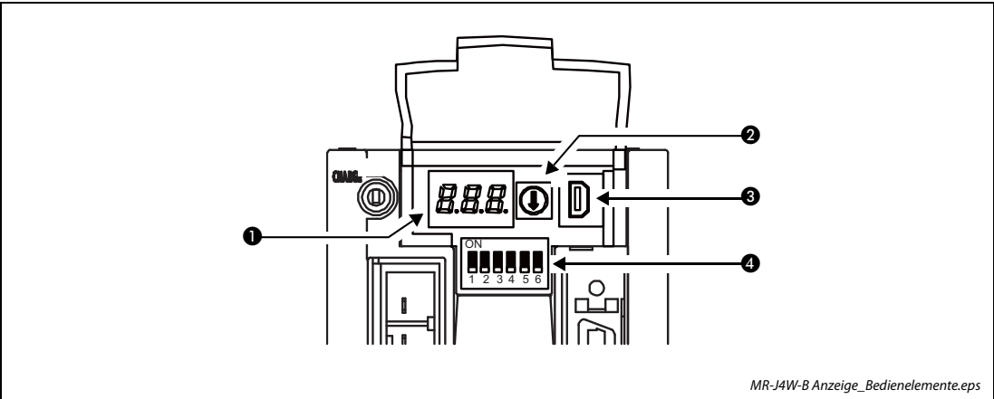
Рис. 6-21: Индикация и выключатели сервоусилителей MR-J4-B
