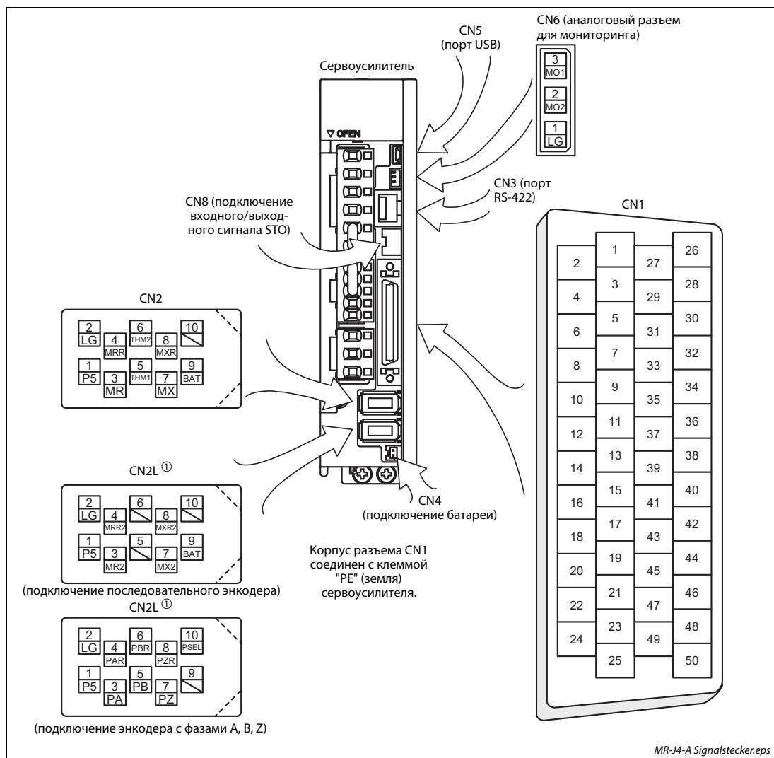
Рис. 4-3: Сигнальные выводы MR-J4-A
