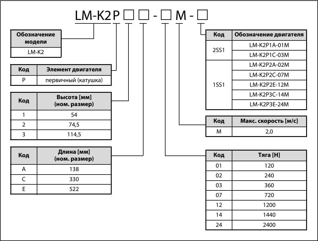
Рис. 3-22: Обозначение серводвигателей серии LM-K2 (первичный элемент – катушка)
