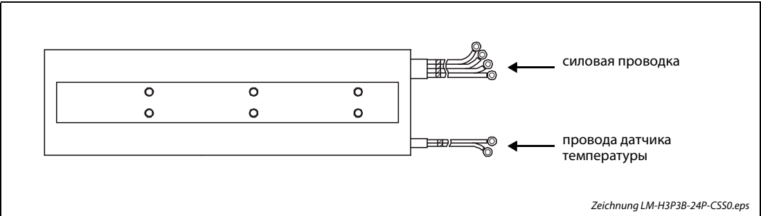
Рис. 3-16: Серводвигатели серии LM-H3 (первичный элемент – катушка)
