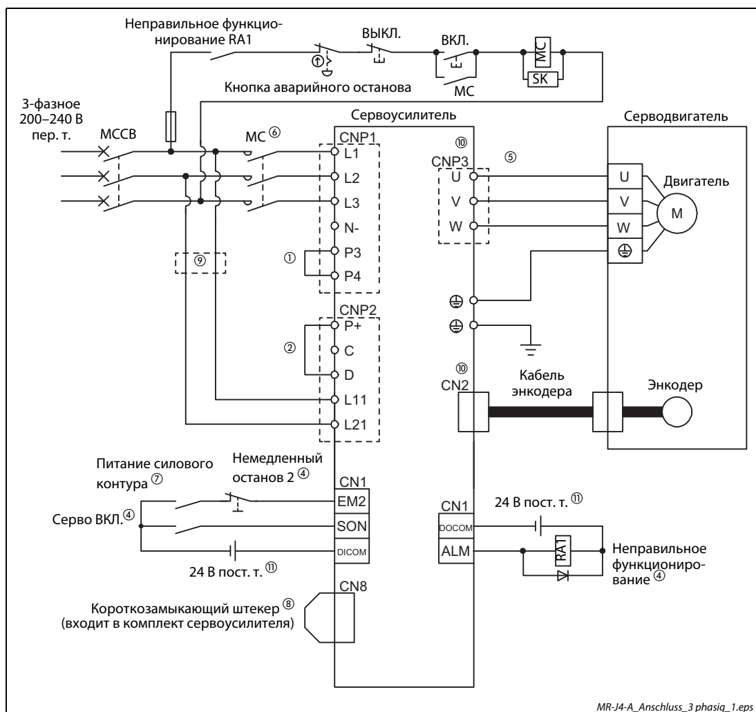
Рис. 4-27: Подключение сервоусилителей MR-J4-10A(-RJ)...MR-J4-350A(-RJ)
