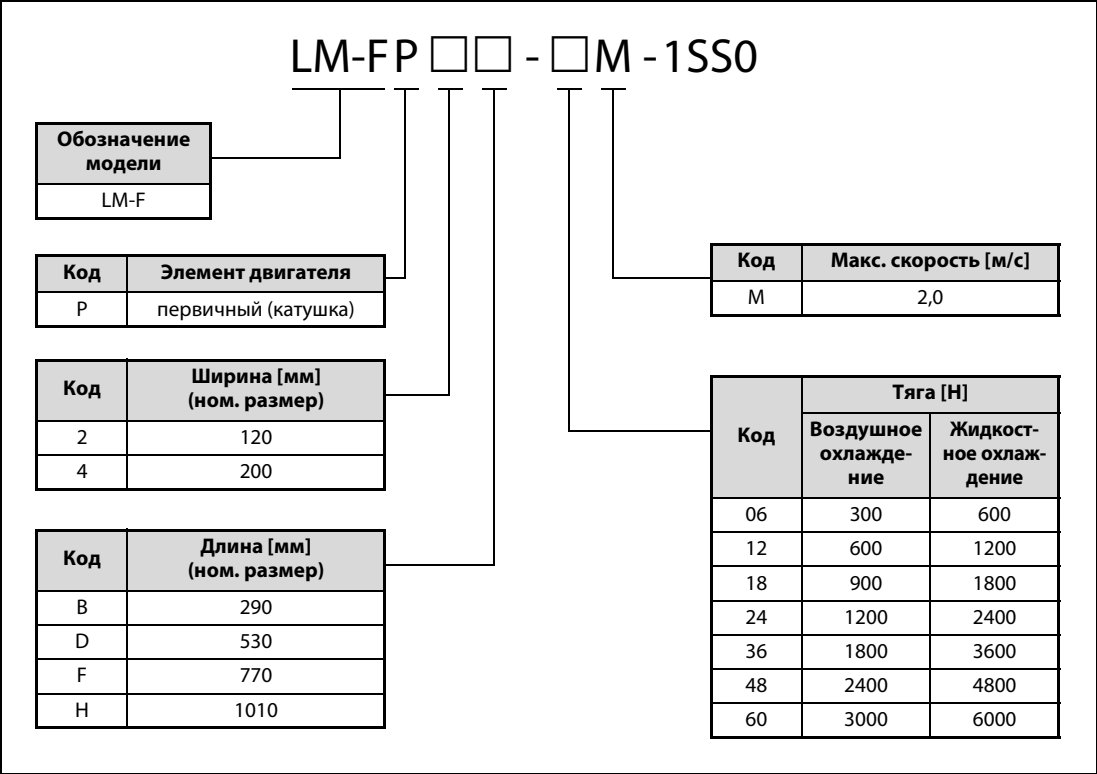
Рис. 3-20: Обозначение серводвигателей серий LM-F (первичный элемент – катушка)
