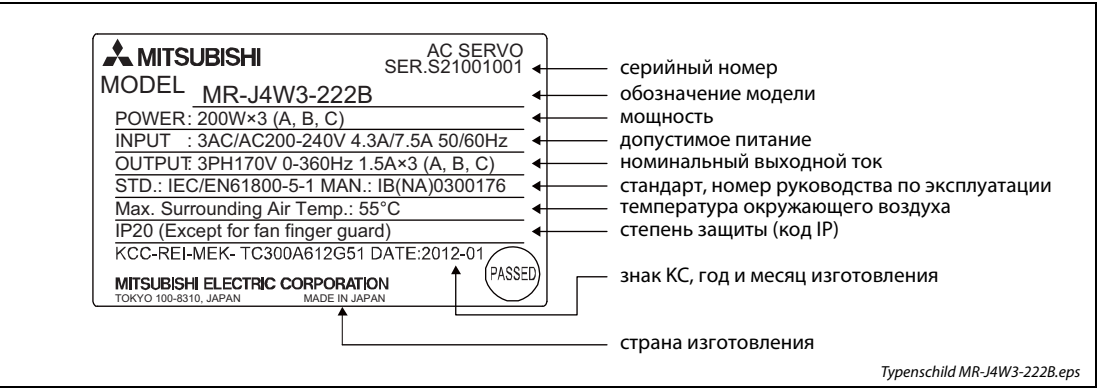
Рис. 2-13: Табличка данных MR-J4W3-222B
